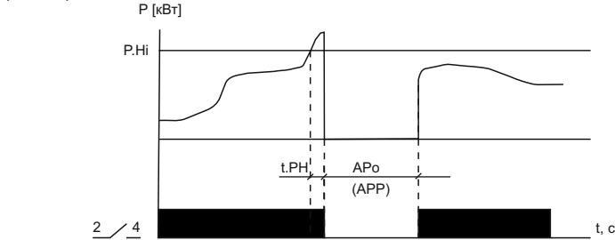
Диаграмма работы реле мощности
